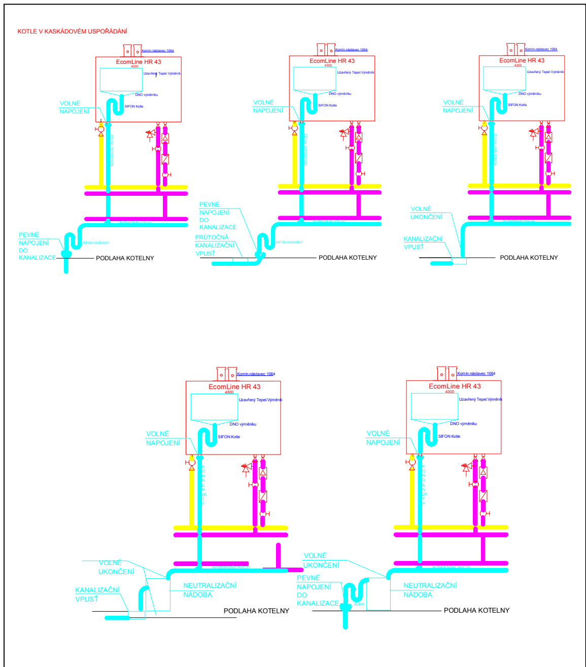
Obr. 3 Příklady připojení kondenzátních potrubí u kotlových kaskád.
