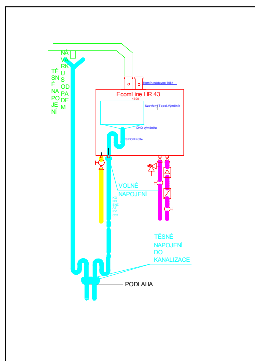
Obr. 2 Princip svádění kondenzátů od kotle a z kouřovodu.
